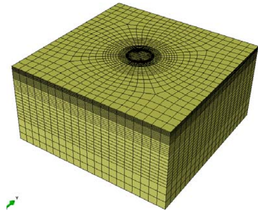
Fig. 2 FEM Mesh
