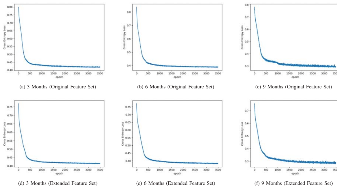
Fig. 2 Loss values
