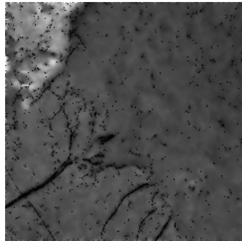
(d) NormalShrink
