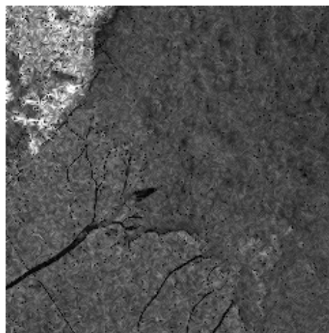
(f) KalmanShrink
