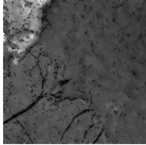
(b) VisuShrink
